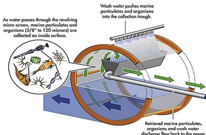
شکل ۳: شماتیک آشغالگیرهای استوانه‌ای
