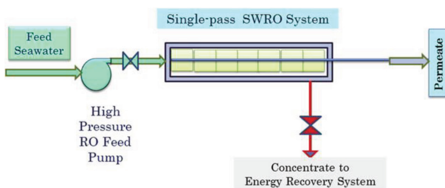
شکل ۴: سیستم SWRO تک گذر
