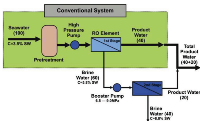
شکل ۷: سیستم SWRO دو مرحله‌ای
